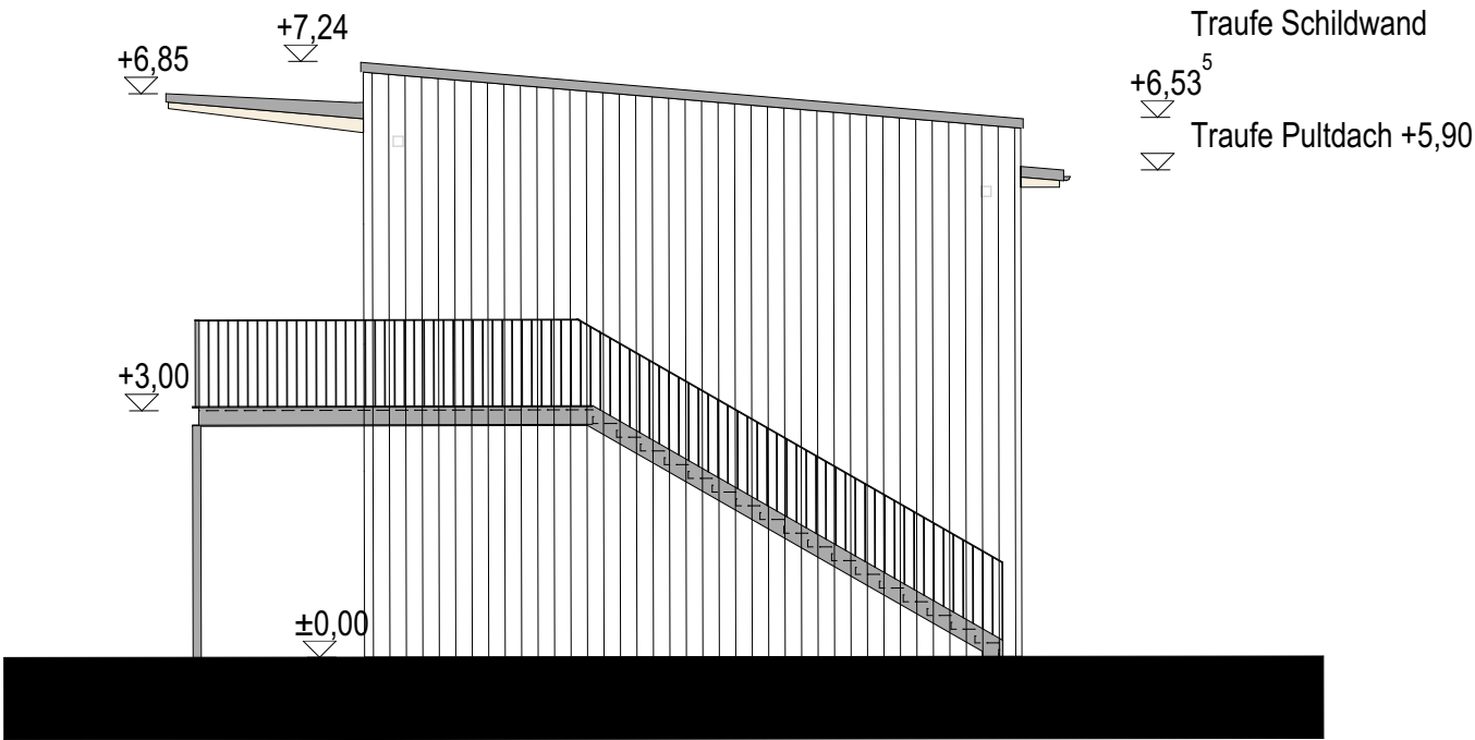
Ansicht N-O
