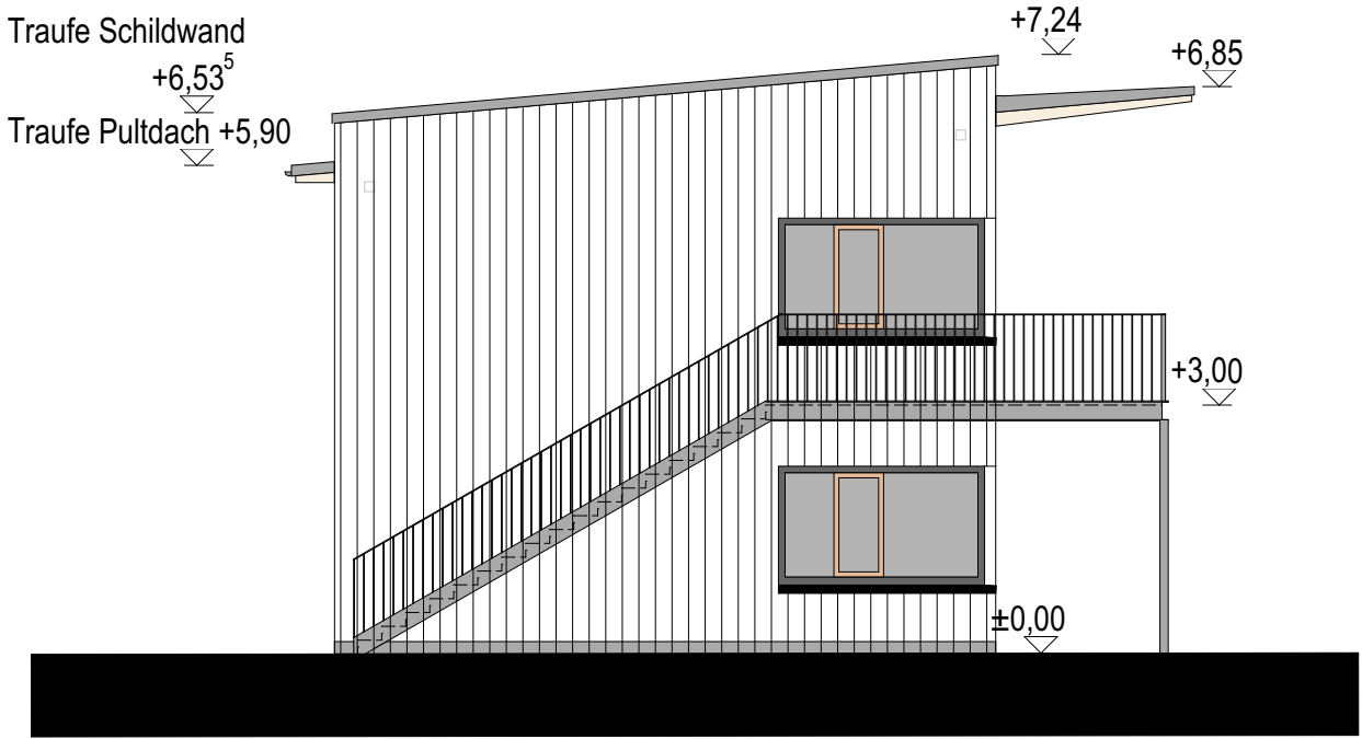
Ansicht S-W
